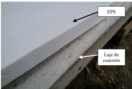
Fig. 3. Revestimento de EPS sendo colado à face superior da laje de concreto.
