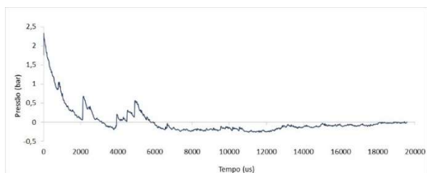
Fig. 1. Diagrama de pressão gerado por um sensor piezoelétrico [11].
