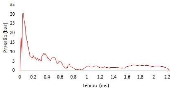
Fig. 4. Diagrama de pressão com registro de pico de pressão refletida no experimento 3.
