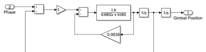
Fig. 5. Tracking loop.
